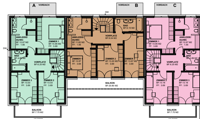
OBERGESCHOSS A / B / C
