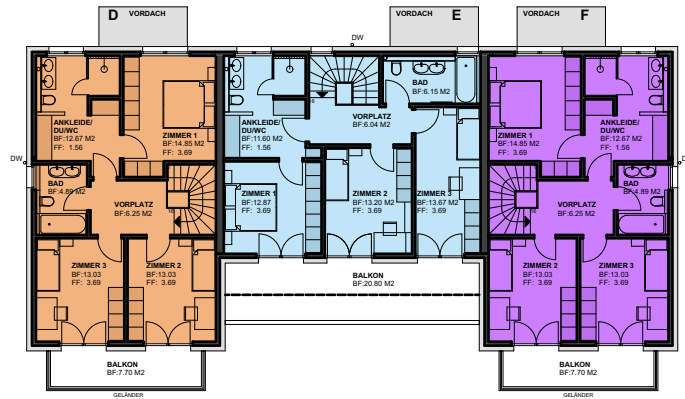
OBERGESCHOSS D / E / F
