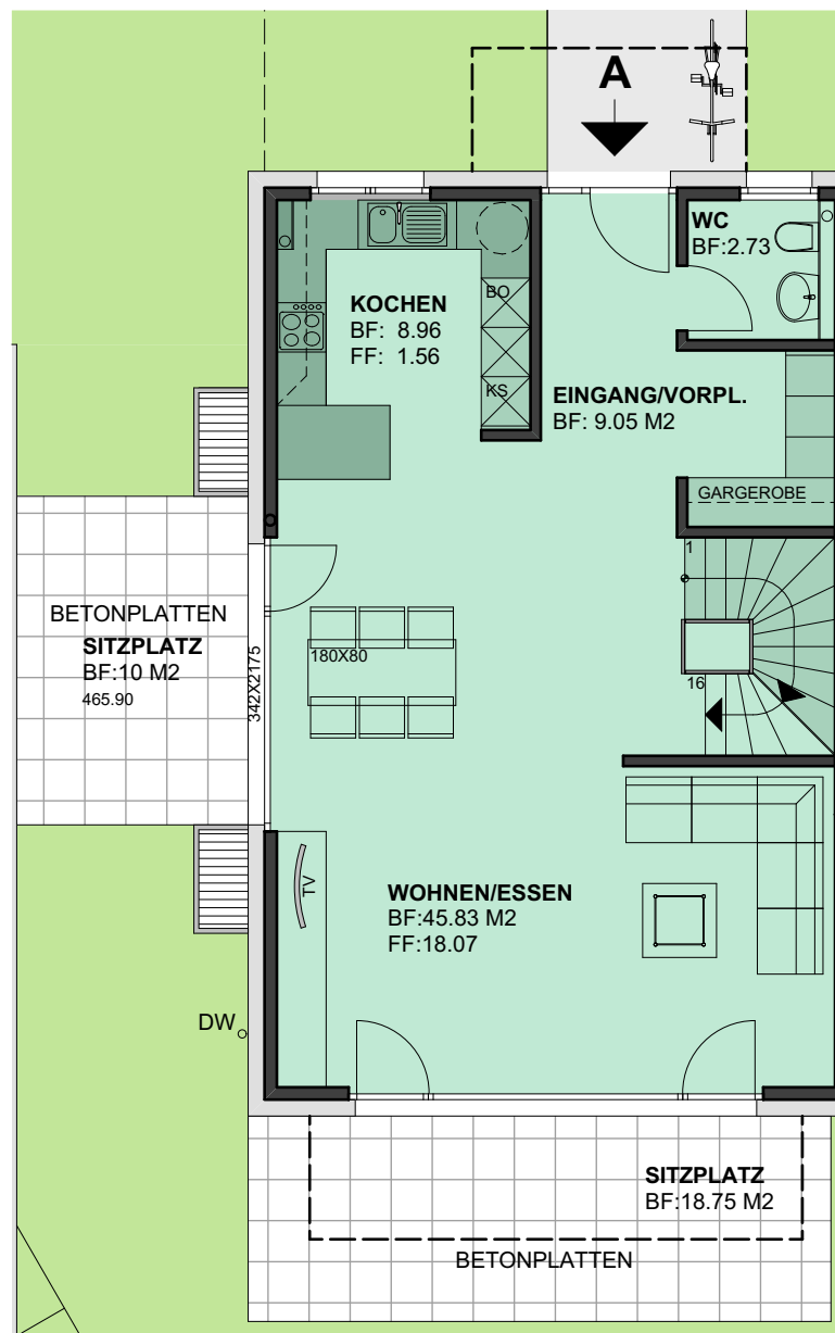
ERDGESCHOSS
