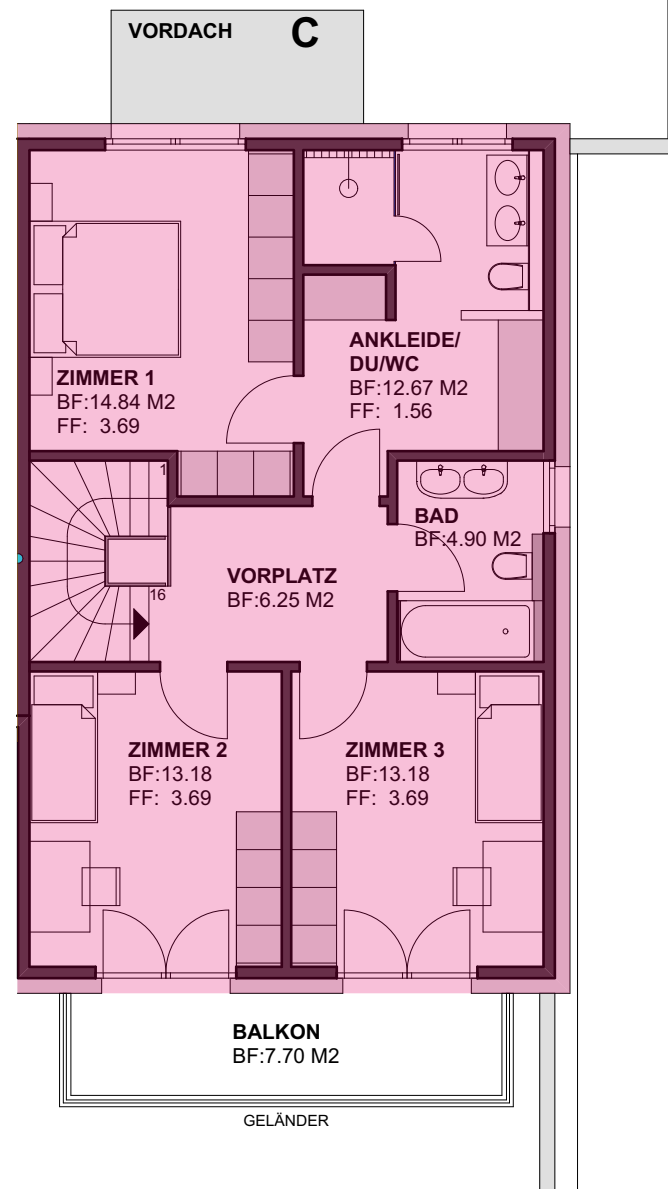
OBERGESCHOSS
